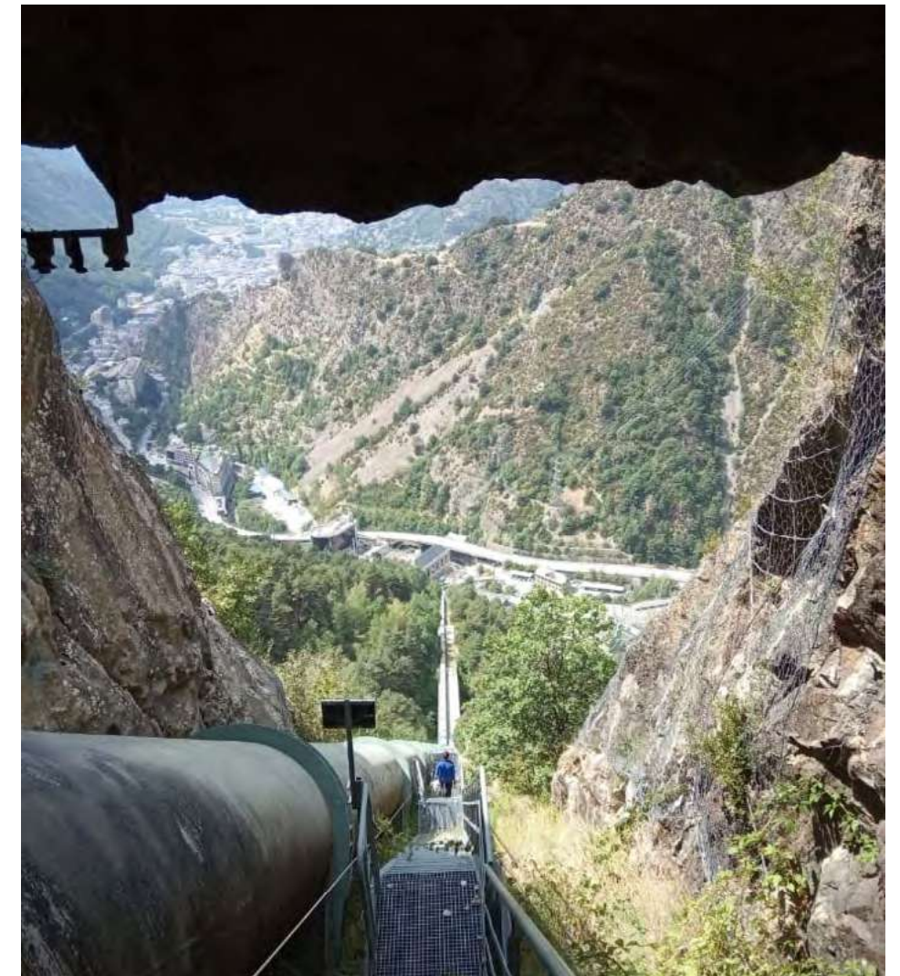
Manteniment de la canonada forçada de la Central hidroelèctrica.
