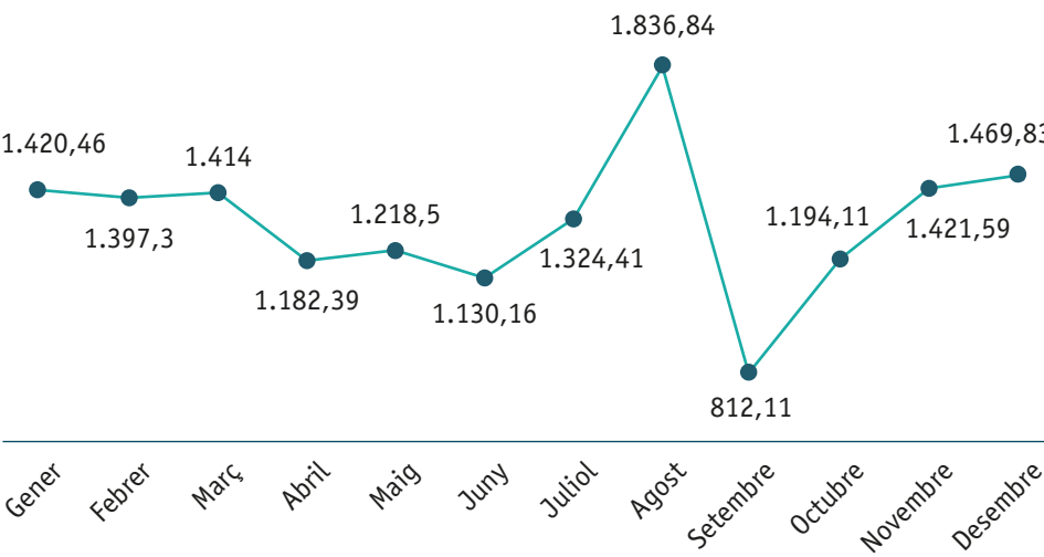
PRODUCCIÓ MENSUAL DEL CENTRE DE TRACTAMENT DE RESIDUS D'ANDORRA (MWh)
